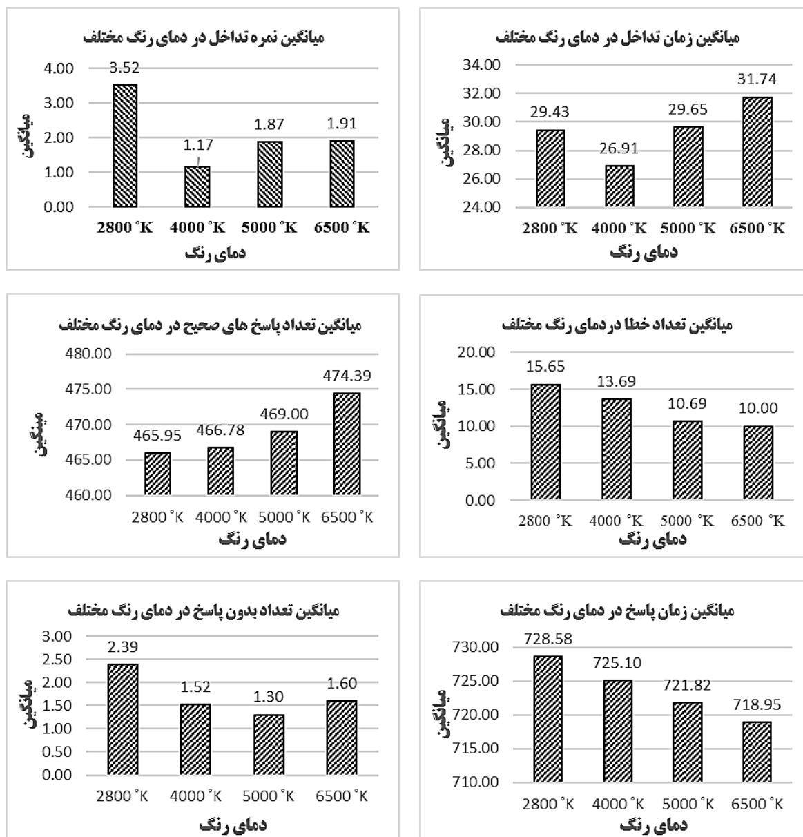
شکل ۳- مقایسه میانگین نمره تداخل، زمان تداخل، پاسخ های صحیح، تعداد خطا و متوسط زمان پاسخ در سیستم های روشنایی با دمای رنگ مختلف
